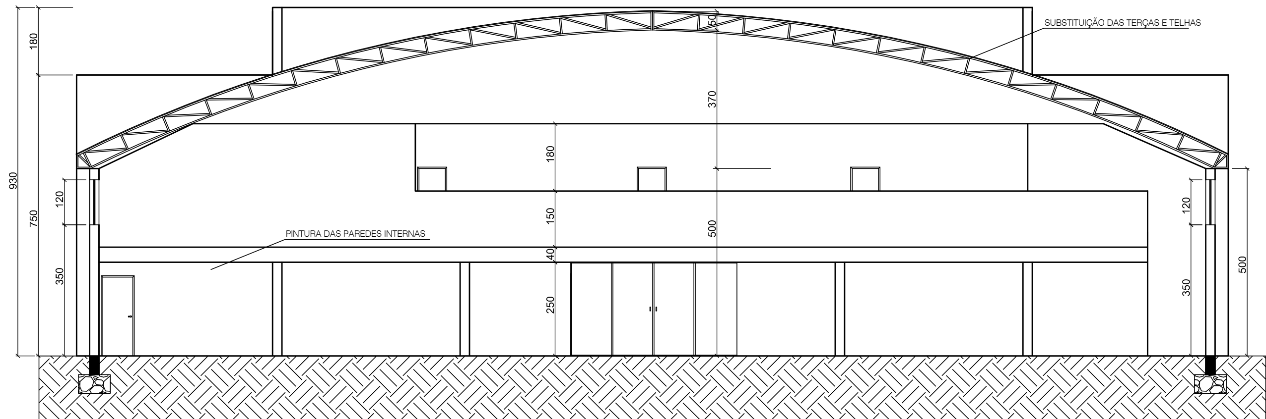
— ARQ CORTE TRANSVERSAL A-A' ESC: 1/100
