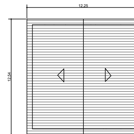
02 PLANTA COBERTURA ESC: 1/750
