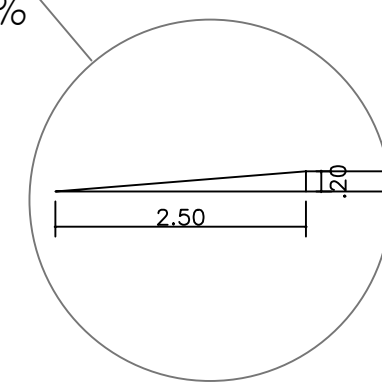
DETALHE RAMPA
