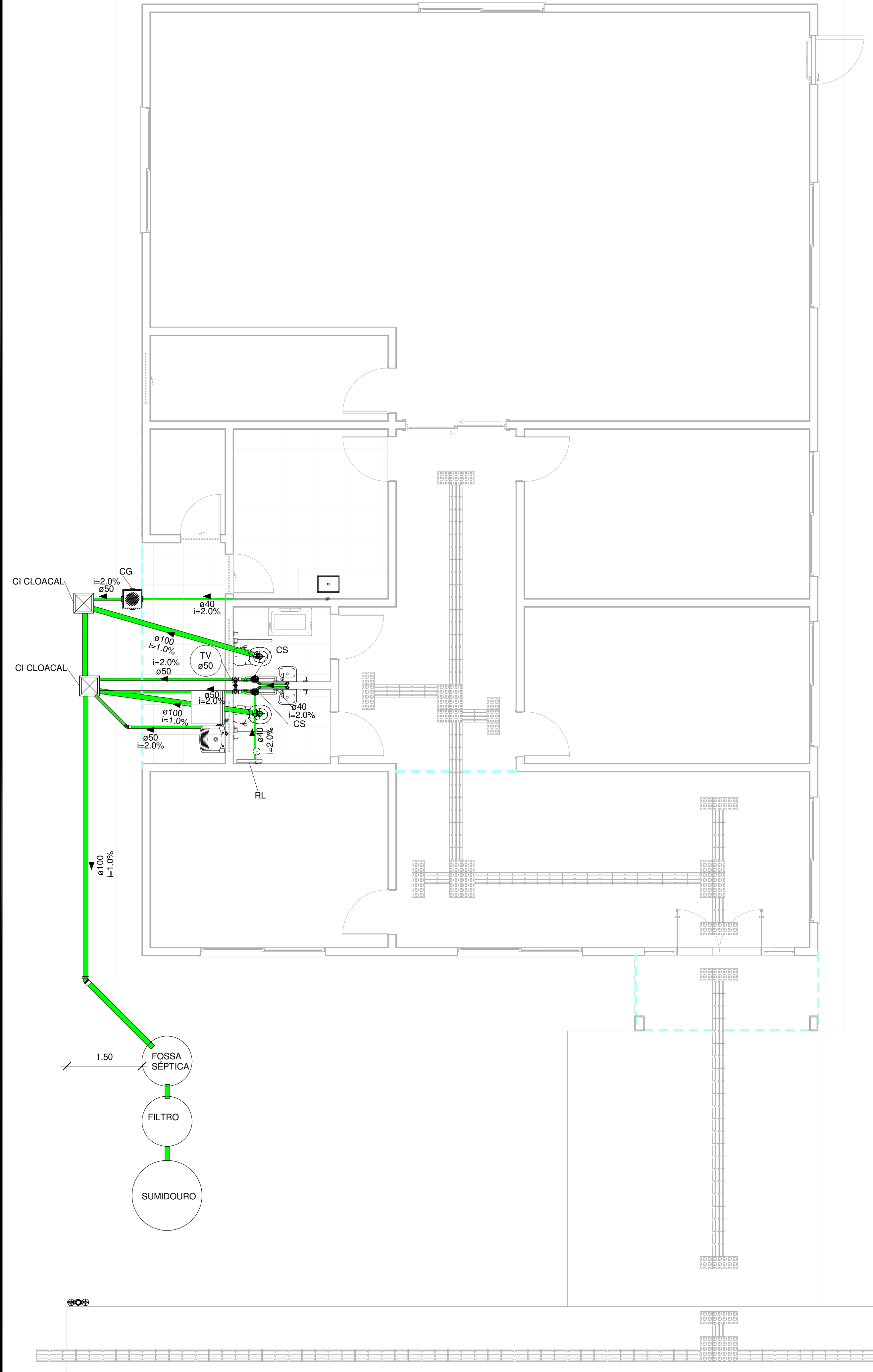
1 PLANTA ESGOTO 1:50
