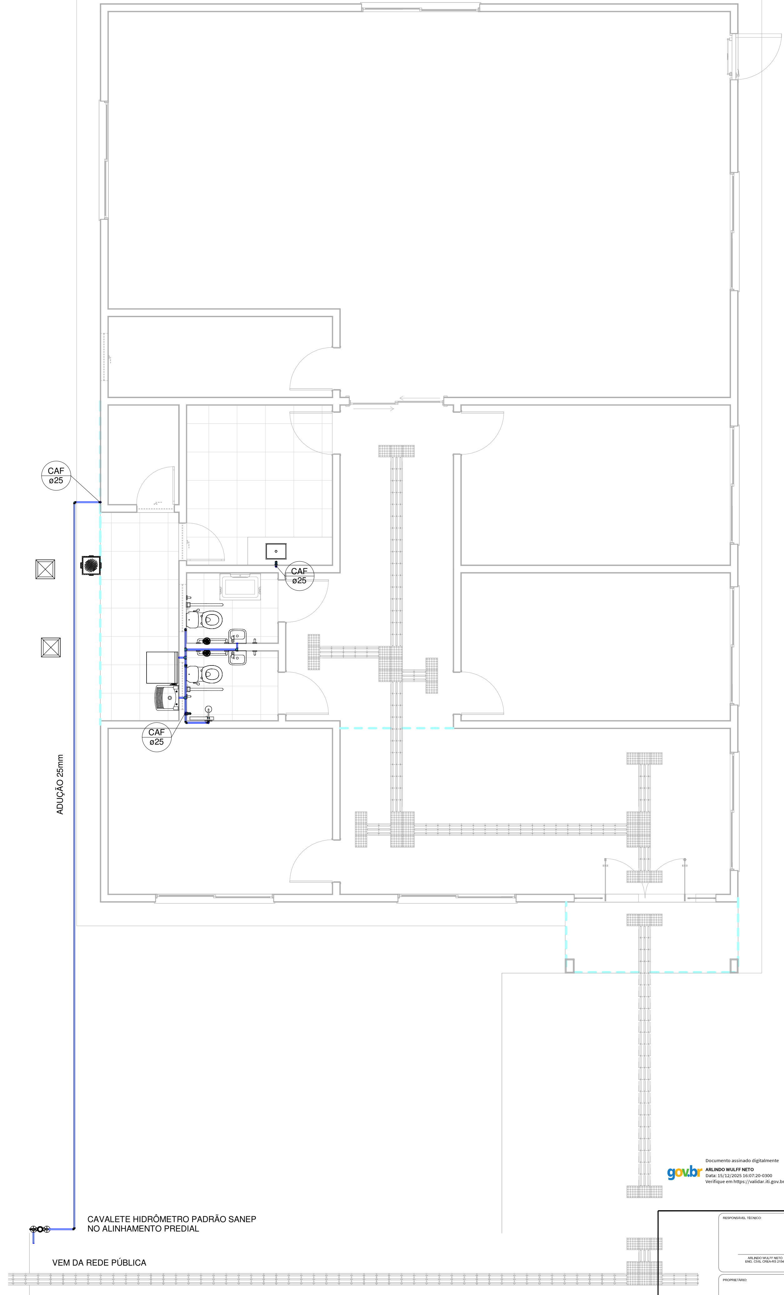
2 PLANTA ÁGUA FRIA - ALIMENTAÇÃO 1:50
