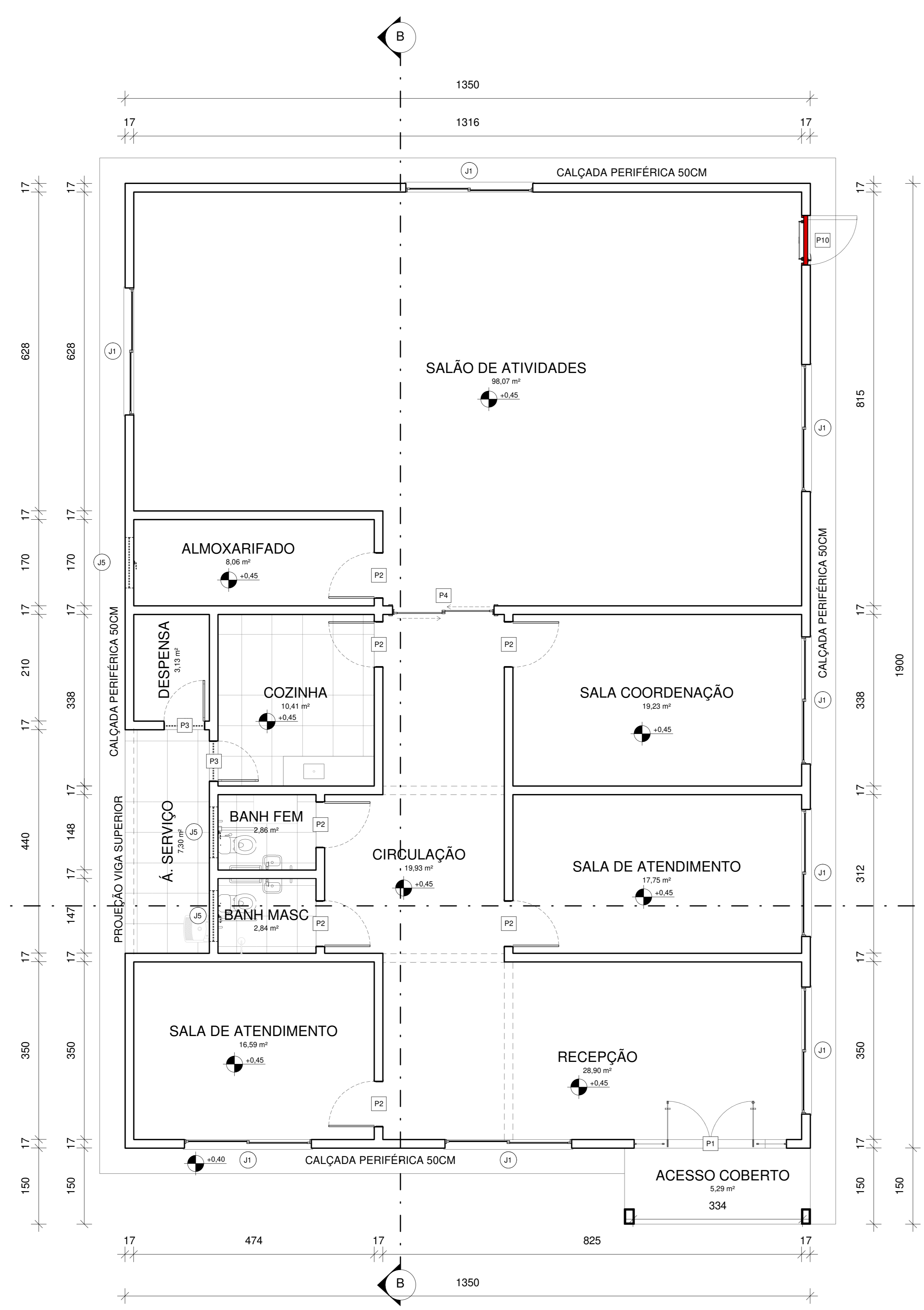
1 PLANTA BAIXA - TÉRREO Escala: 1 : 50
