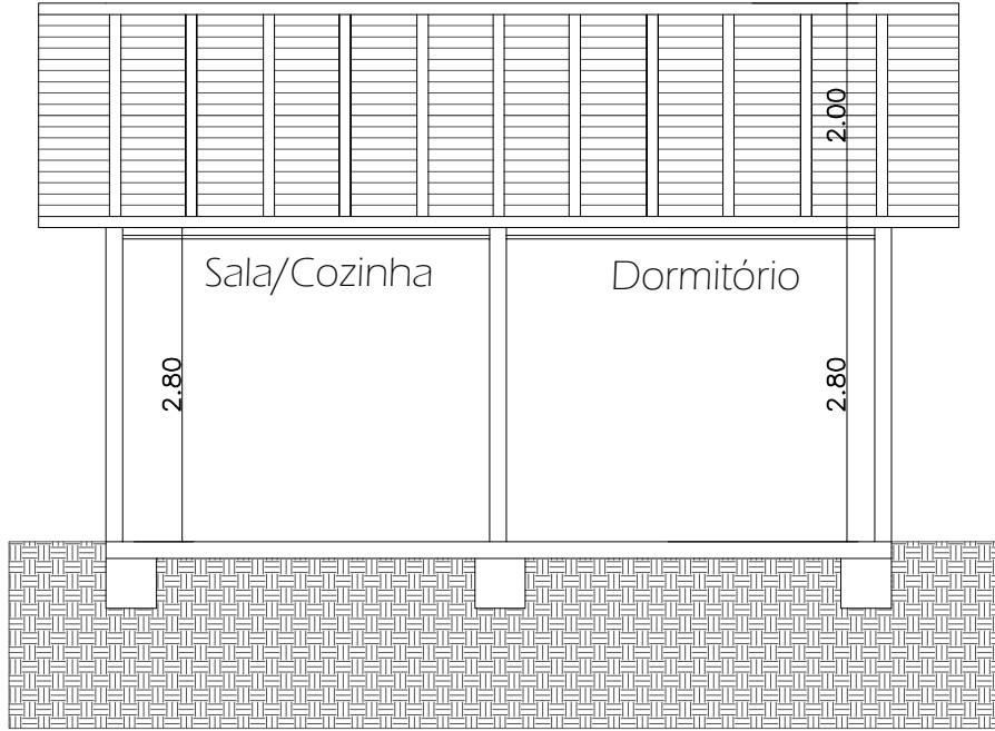
01 Corte A-A ESC: 1/75
